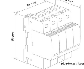
4 Poles
