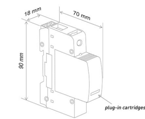
1 Pole
