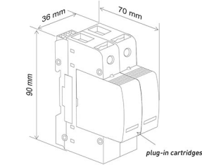
2 Poles
