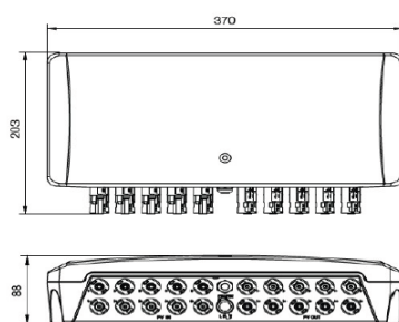
Strings: 3,4 or 5
